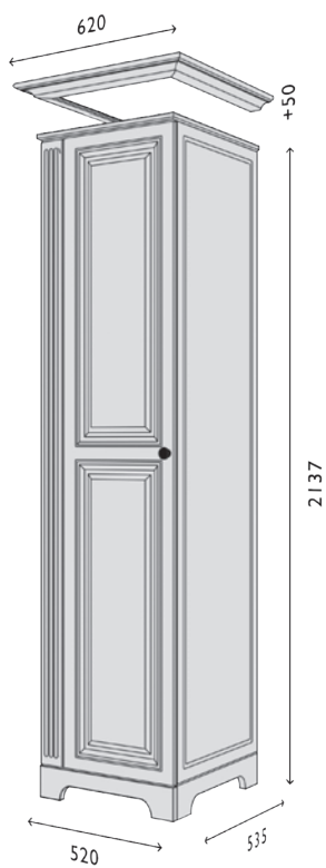
Схема Пенал фасад-V2 декор «Мадрид модуль-1».
