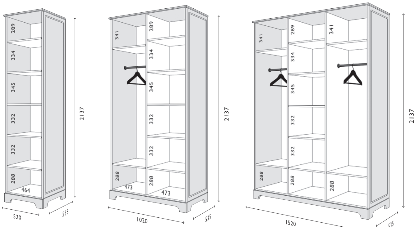
Схема Пенал без фасаду «Мадрид модуль-1».
