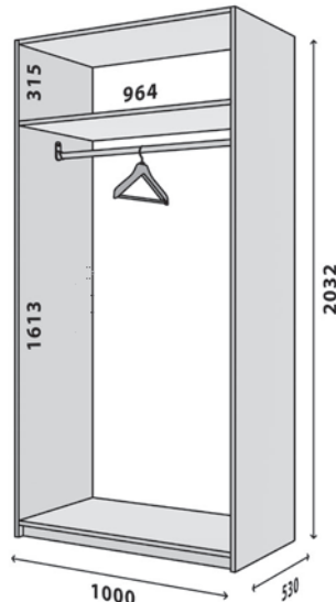
Модуль М-2 УНІ ШУ-1000х2050 Фасад-500х2015 (2 шт.)
