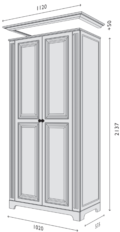
Схема Шафа фасад-V2 декор «Мадрид модуль-2».
