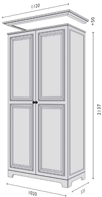
Схема Шафа фасад-V2 «Мадрид модуль-2».
