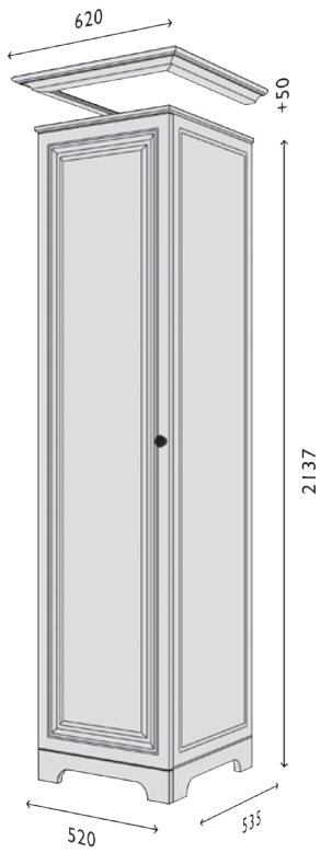
Схема Пенал фасад-V1 «Мадрид модуль-1».
